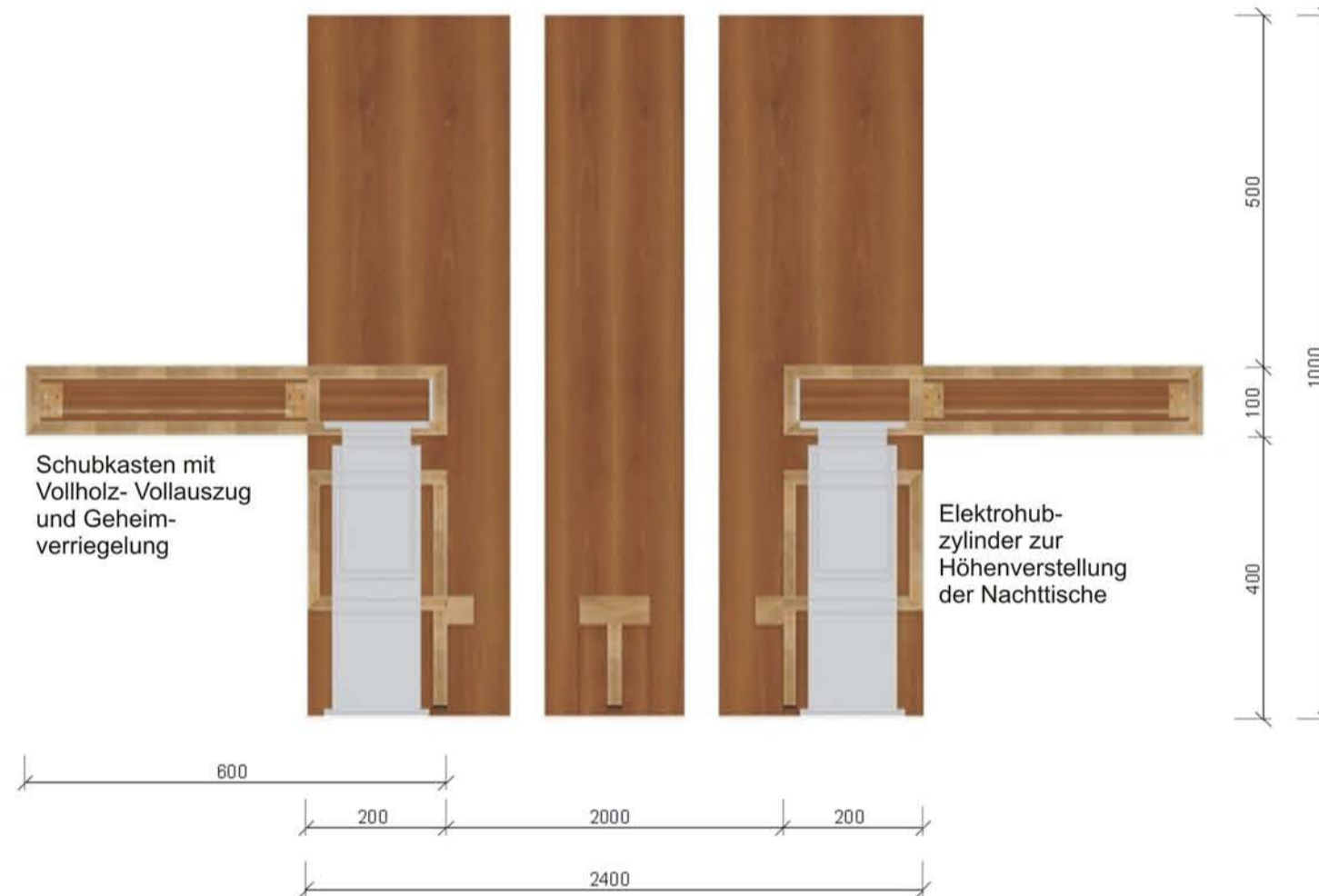
Schnitt C-C
