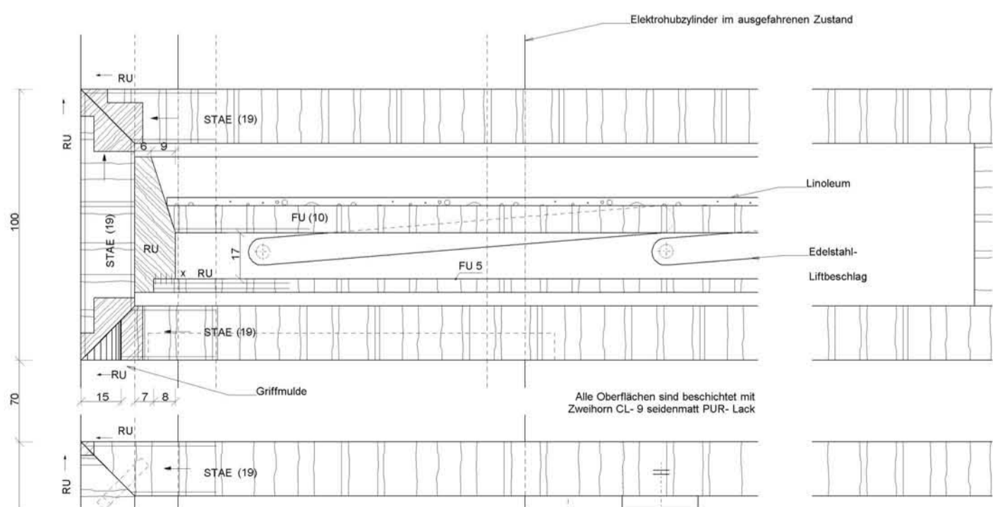
Detail: Schubkasten der Sitzbank mit Liftbeschlag
