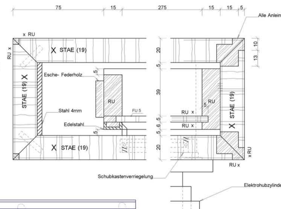
Detail: Verriegelung des Schubkasten am Nachttisch
