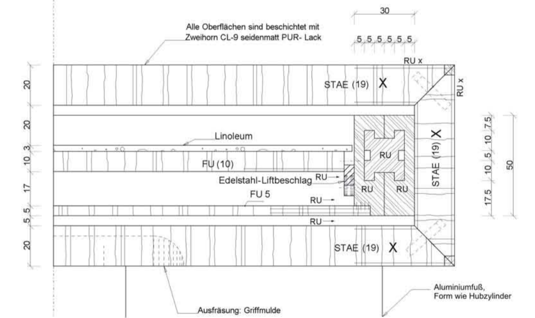
Detail: Vollholz- Vollauszug
