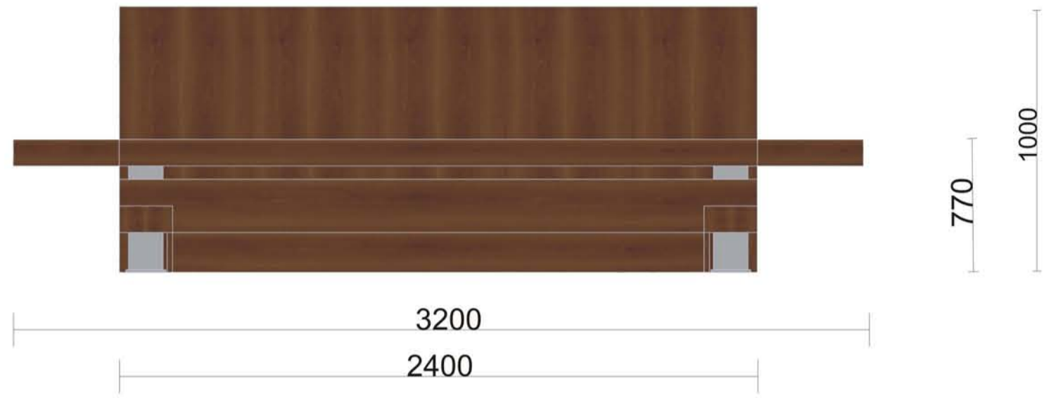
Draufsicht
